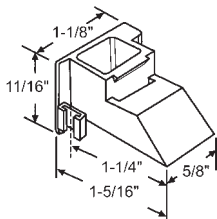
900-9963 LH & RH Set
