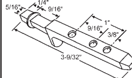
85-5003 Die Cast SIMONTON
