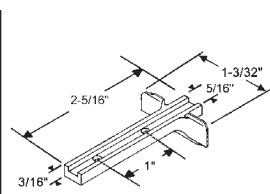
85-718 Die Cast SILVERLINE
