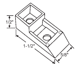
900-10122-OS Nylon KINCO
