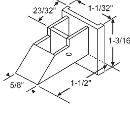
60-652A LH & RH Set ALSCO/ANACONDA
