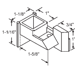
60-666 LH & RH Set. Black MANNIX
